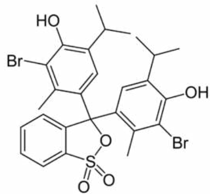
أزرق البروموتيمول
