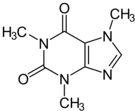
الكافيين
